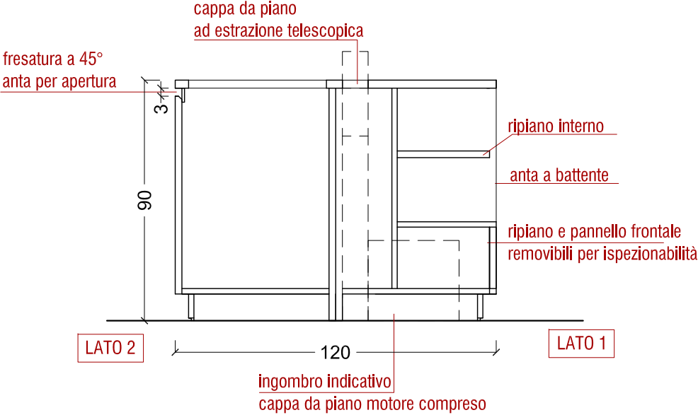
DETTAGLIO CUCINA CON CAPPDA PIANO AD ESTRAZIONE TELESCOPICA
