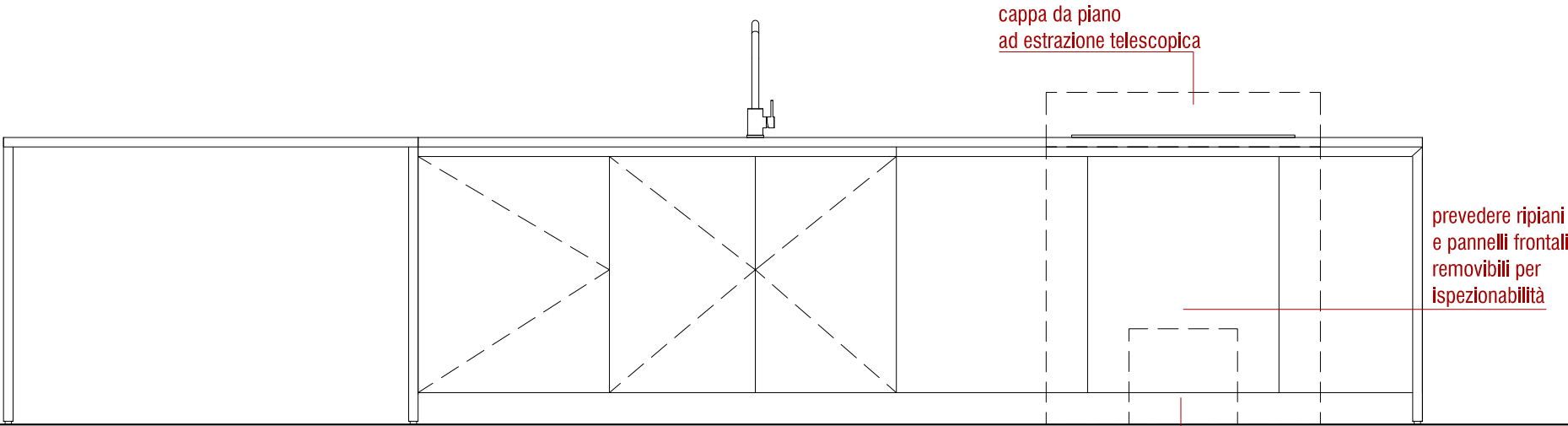
PROSPETTO LATO 1
